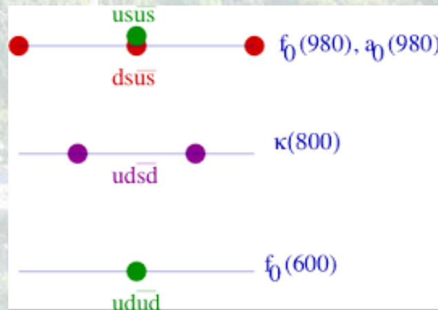
Виявлені невідомі "екзотичні мезони" - раніше невідомі субатомні частинки (1997)
